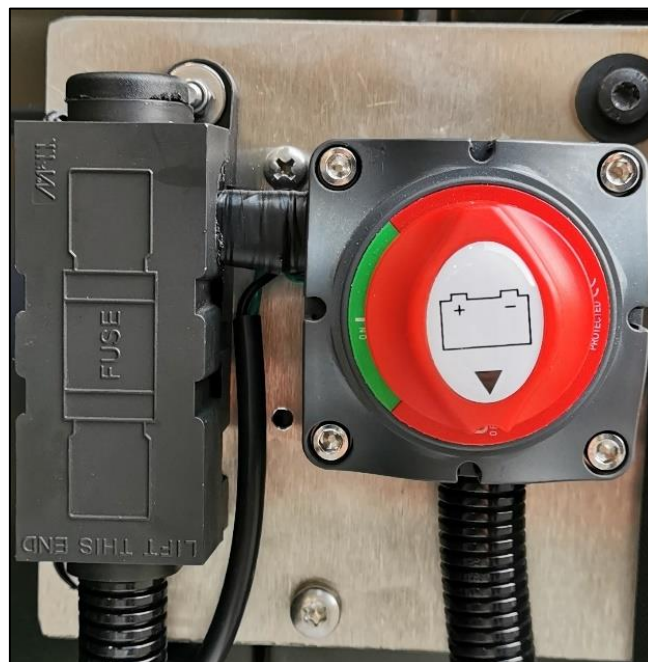
Abbildung 2: Hauptschalter; Zustand im Bild: AUS (Abbildung kann abweichend sein)
