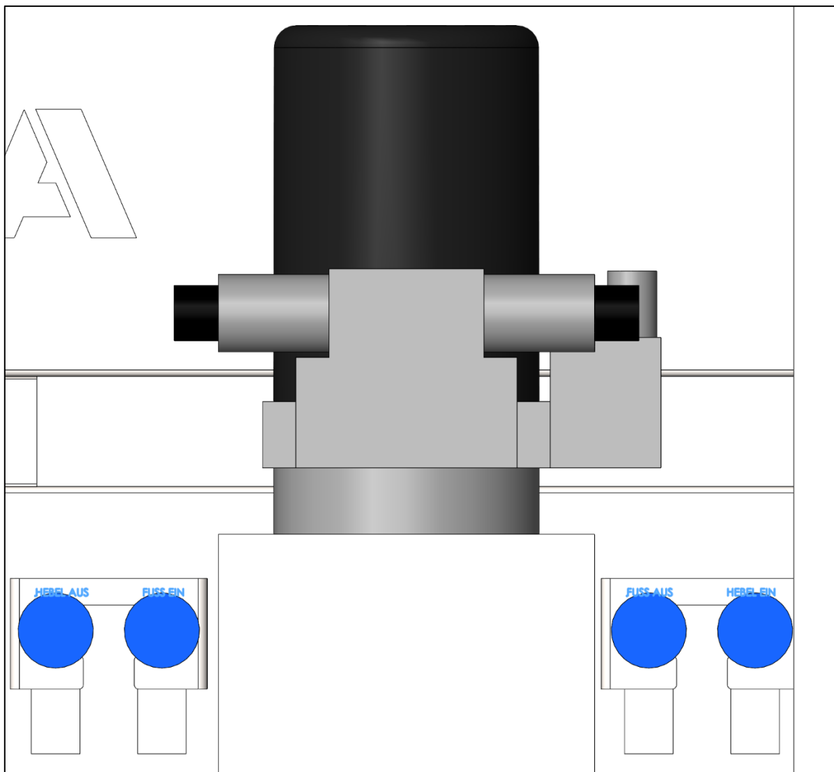
Abbildung 11: Hydraulikaggregat und Hydraulikdrosseln zur Einstellung des Bewegungsablaufes
